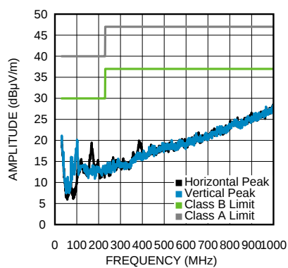
Radiated EMI (EN 55022) V_{IN} = 12V , V_{OUT} = 5V , I_{OUT} = 8A
